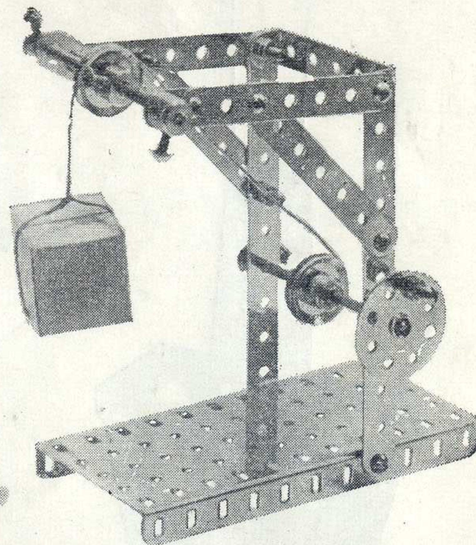
Csörlős emelő
