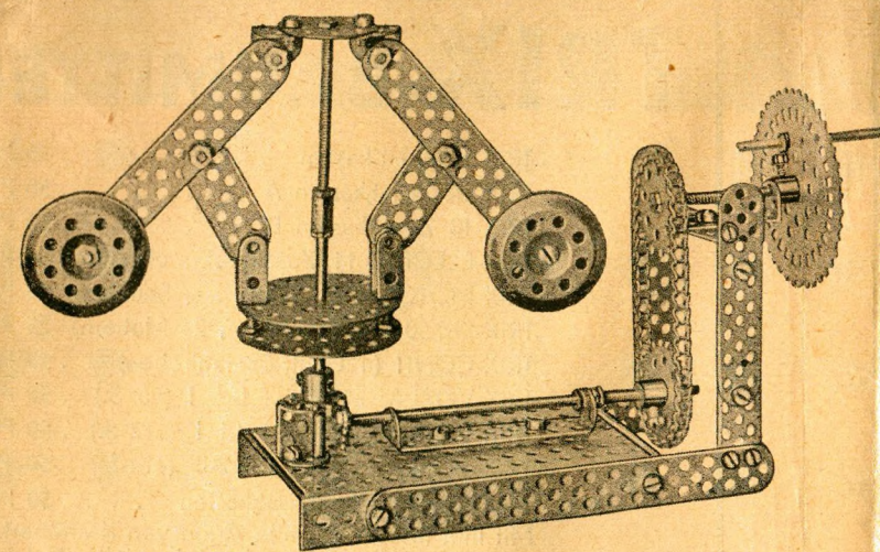
Regulator-Modell zur Darstellung der Fliehkraft. Gebaut mit je 1 Kasten 1, 1a, 1b und 1c
