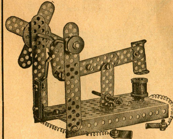
Magnet-Maschine aus TRIX-Electro
