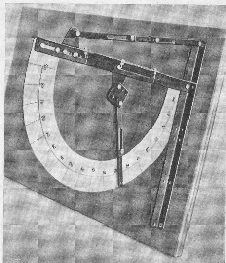
1.65 Indicateur de pente
