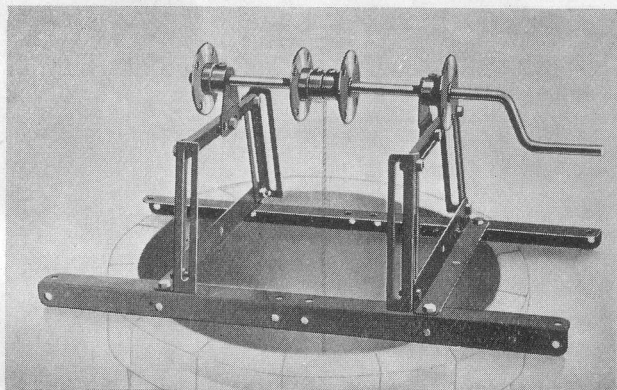
2.67 Treuil de puits
