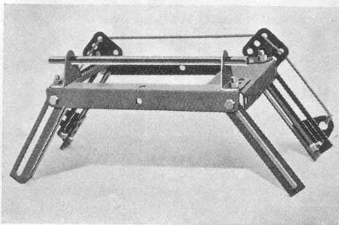
2.52 Etabli de monteur
