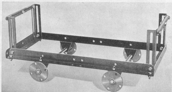
2.75 Chariot à colis
