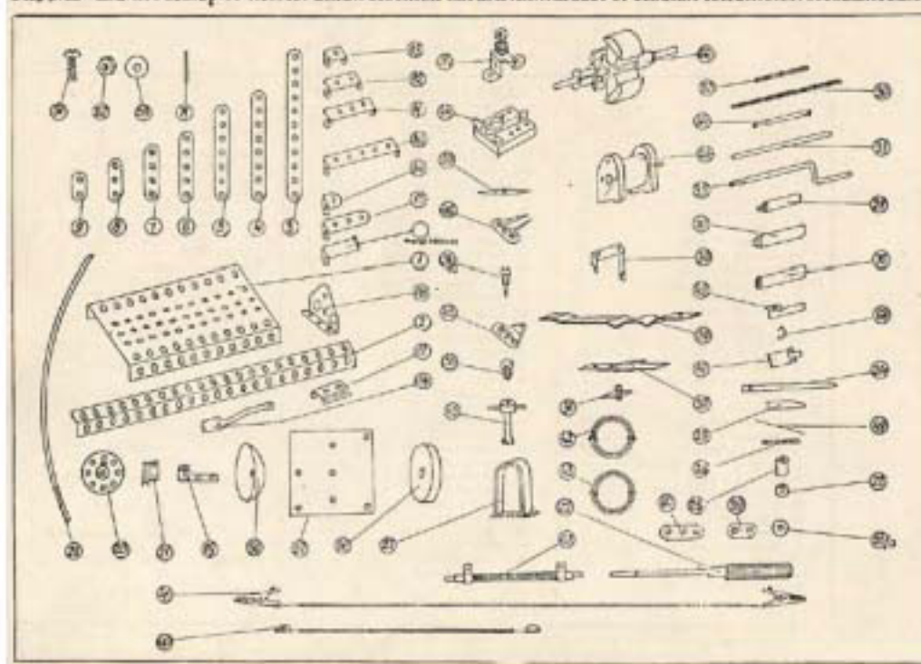
PAJTÁS villamos fémépítő készlet alkatrészeinek ábrái a mintafüzet 3. oldalán feltüntetett sorszámozással
