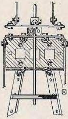
Abb. 209 a Schnitt durch den Kopf des Bockkranes
