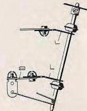
Abb. 212 b Steuerwelle
