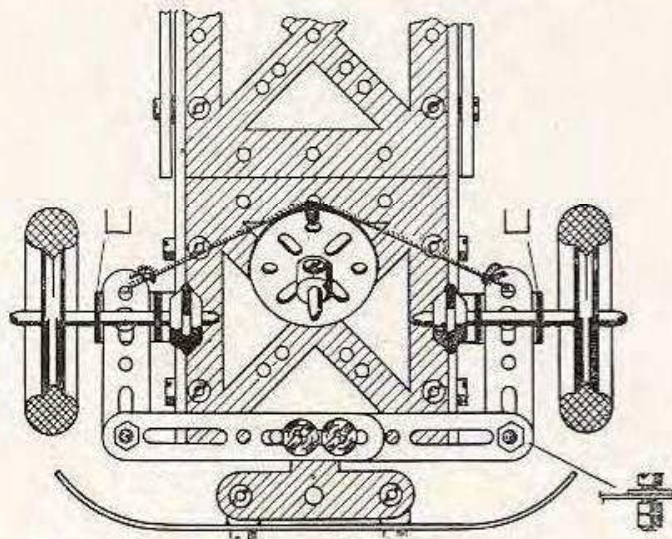
Abb. 74a Unteransicht mit Steuerung des Modelles Nr. 74 auf Seite 25
