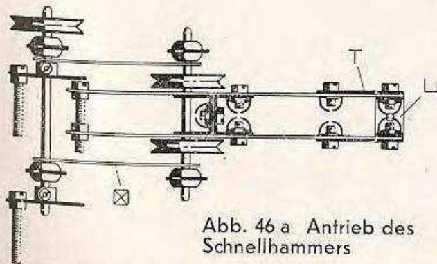
Nr. 46 Schnellhammer
