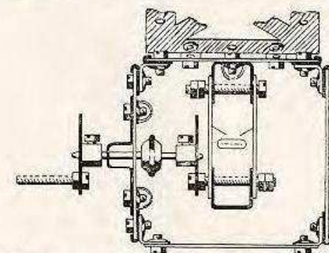
Abb. 45a Schnitt durch den Kurbelantrieb
