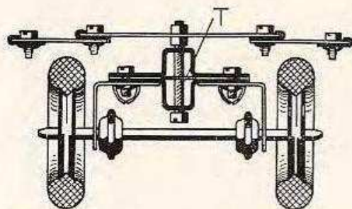
Abb. 70a Lagerung der Vorderachse des Plattenwagens
