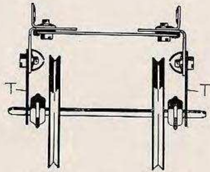
Abb. 201 b Befestigung der mittleren Räder
