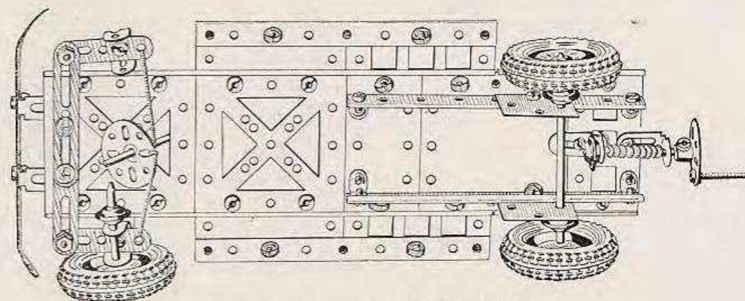
Abb. 207 a Unteransicht des Autos
