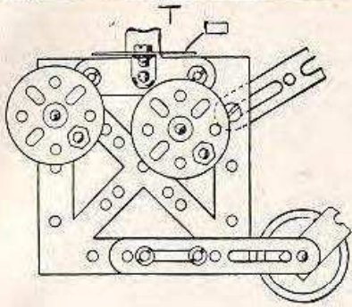
Abb. 50 a Befestigung des beweglichen Auslegerarmes
