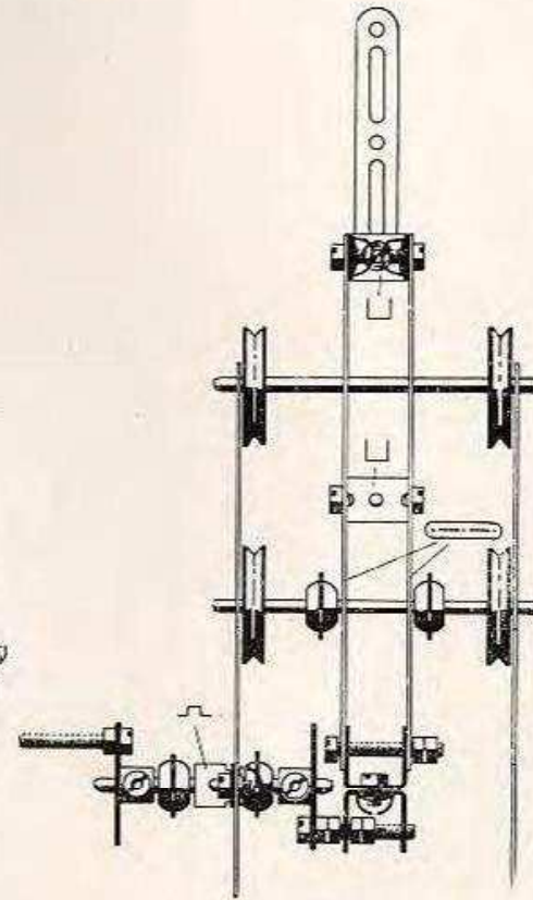
Abb. 47 a Antrieb der Feilmaschine
