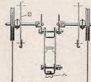
Abb. 214 b Kurbelwelle der Presse
