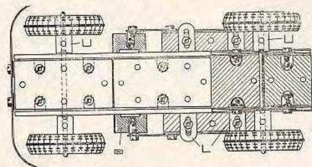
Abb. 58 b Unteransicht des Traktors
