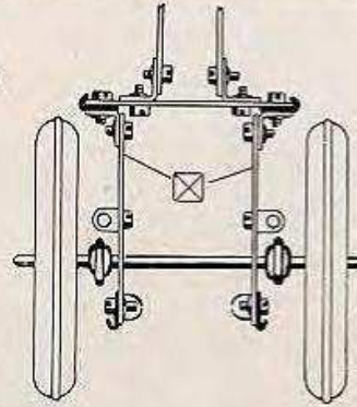
Abb. 204 c Lagerung der Hinterradachse
