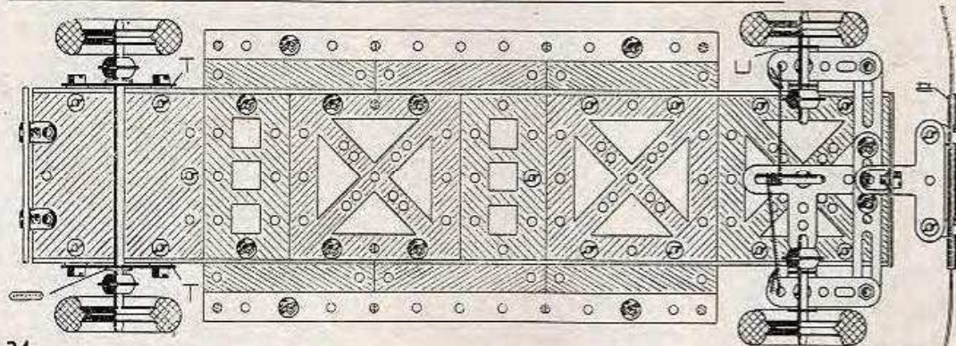
Abb. 205a Unteransicht des Feuerwehrautos
