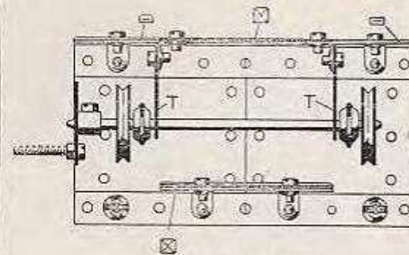
Abb. 214 a Antriebswelle der Exzenterpresse
