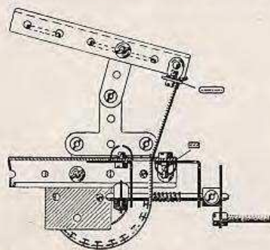
Abb. 207 b Schnitt durch den Seilzug der Feuerwehroleiter
