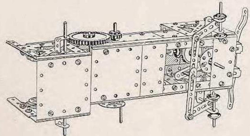
Abb. 302 a Unteransicht
