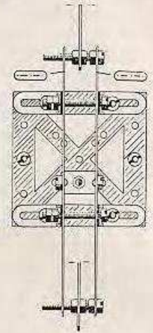
Abb. 221 b Gleitführung der Säge
