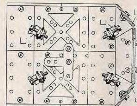
Abb. 301 b Unteransicht des Kranhausbodens
