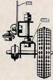
Abb. 204 b Befestigung eines Vorderrades
