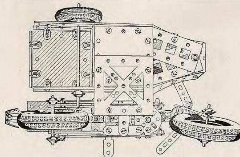
Abb. 218a Unteransicht des Motorrades
