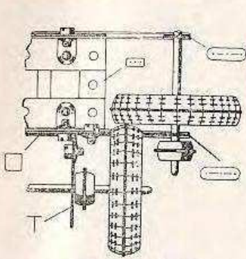
Abb. 55a Antrieb
