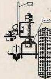
Abb. 74c Befestigung eines Vorderrades
