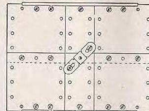
Abb. 301 c Aufsicht auf das Drehgestell
