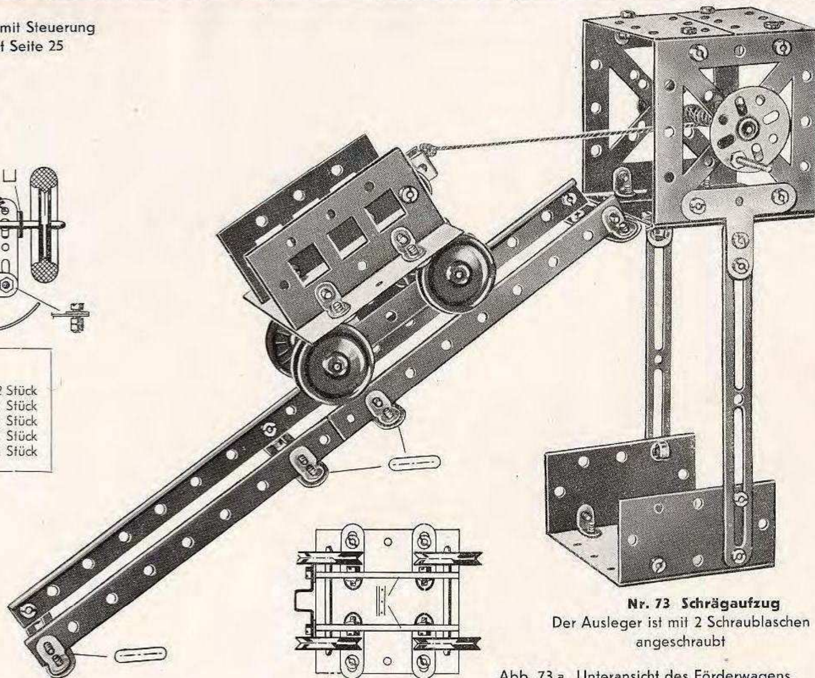
Abb. 73a Unteransicht des Förderwagens
