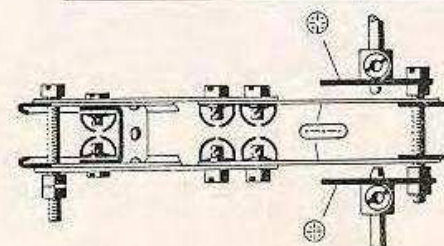
Abb. 66 a Antrieb des Selbstfahrers
