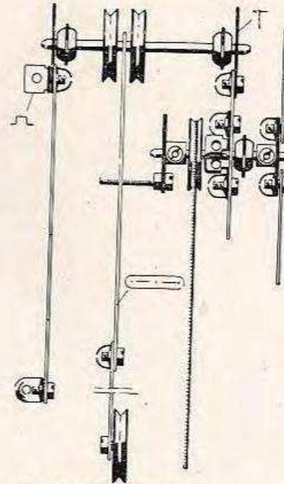
Abb. 56a Schnitt durch die Pendeluhr
