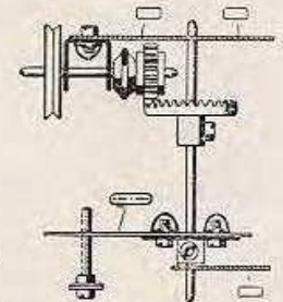
Abb. 302 b Steuerung
