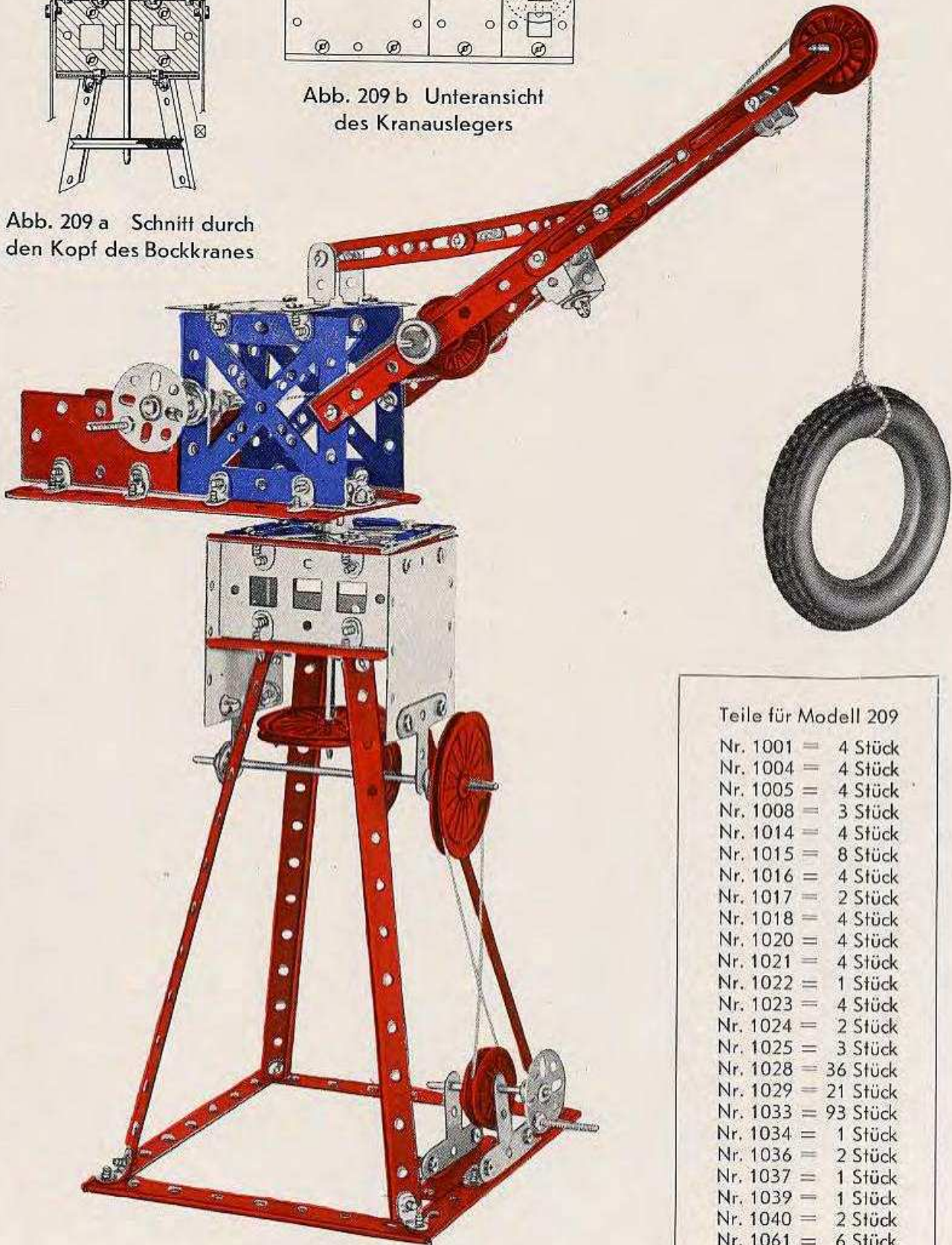
Nr. 209 Bockkran
