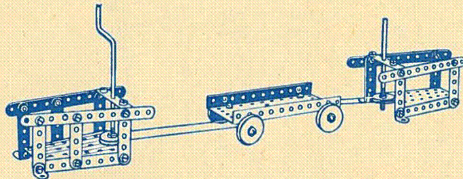
Transportbahn mit endlosem Seil Rope removing van with endless rope Transporteur avec cable sans fin Ferrocarril de transporte de cable sin fin Carrello trasporto a cavo senza fine
