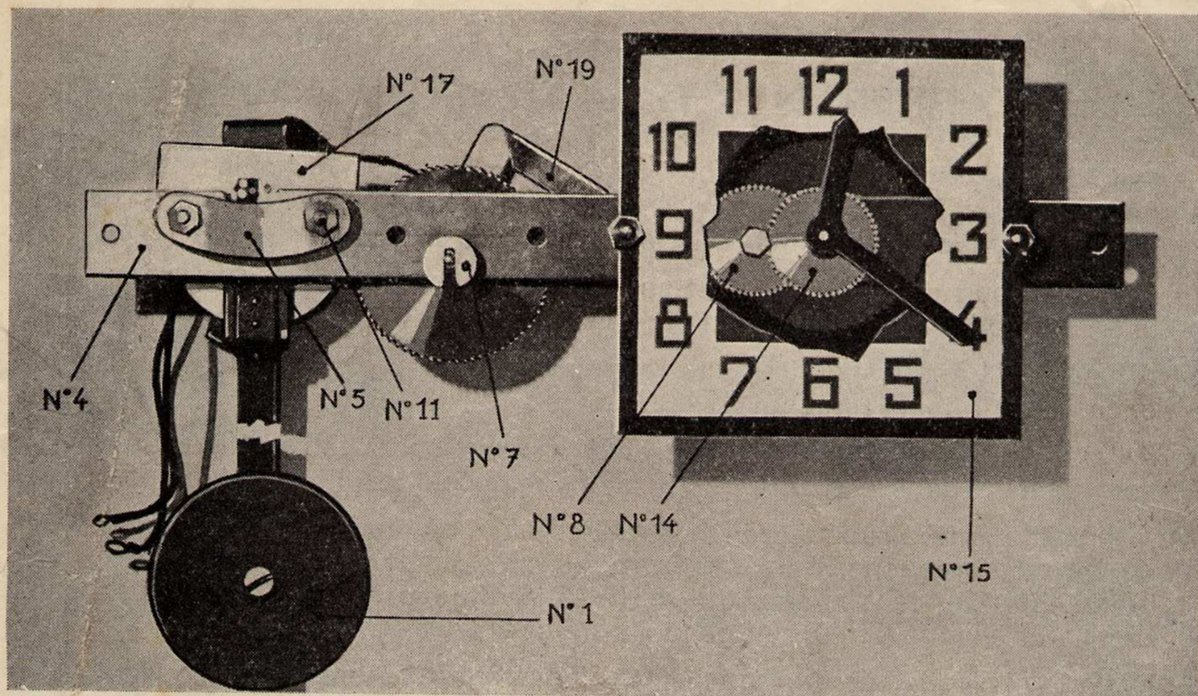
LA PARTIE HORLOGÈRE MONTÉE, VUE DE FACE (N° 20)
