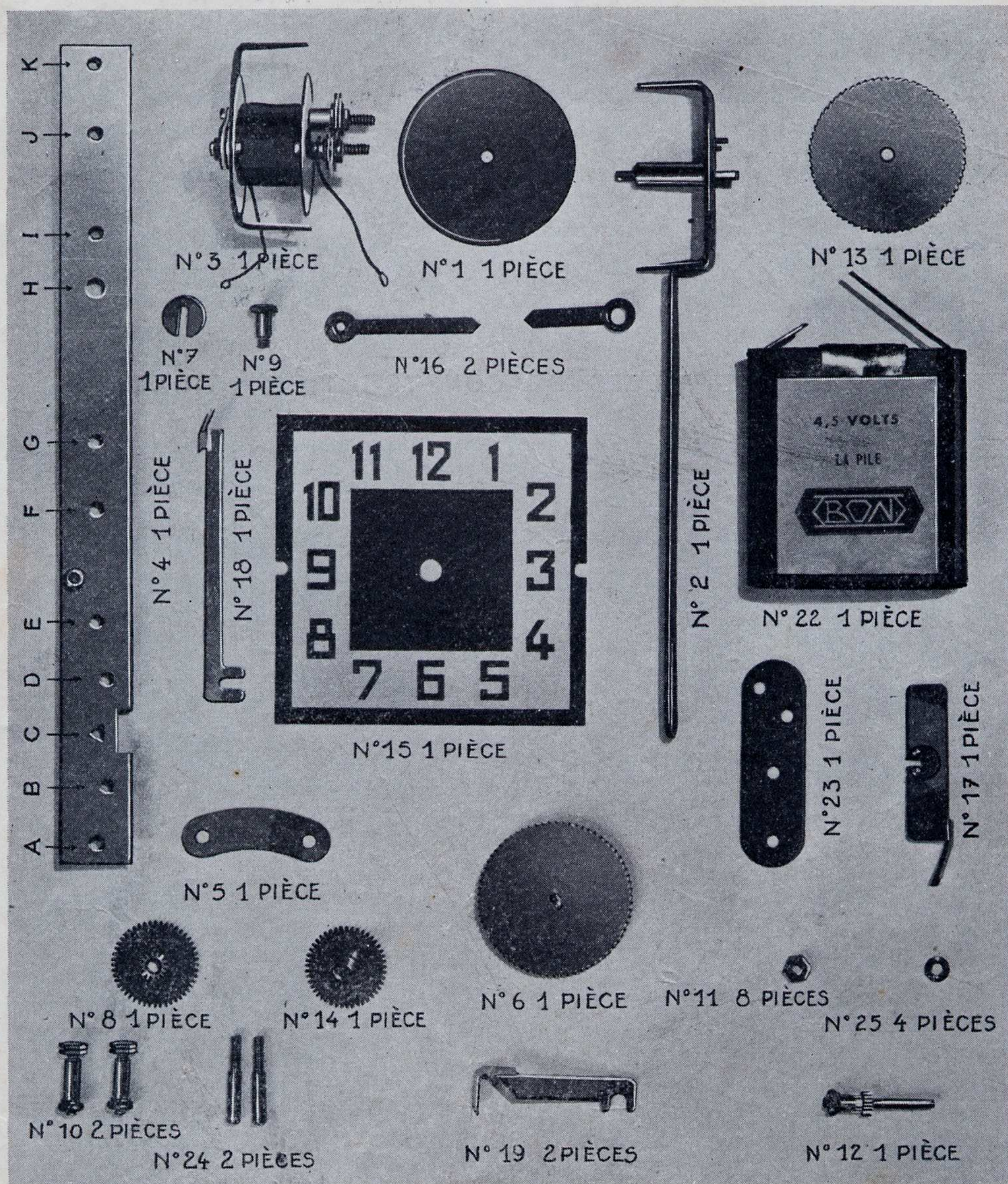
NOMENCLATURE DES PIÈCES DE LA PARTIE HORLOGÈRE
