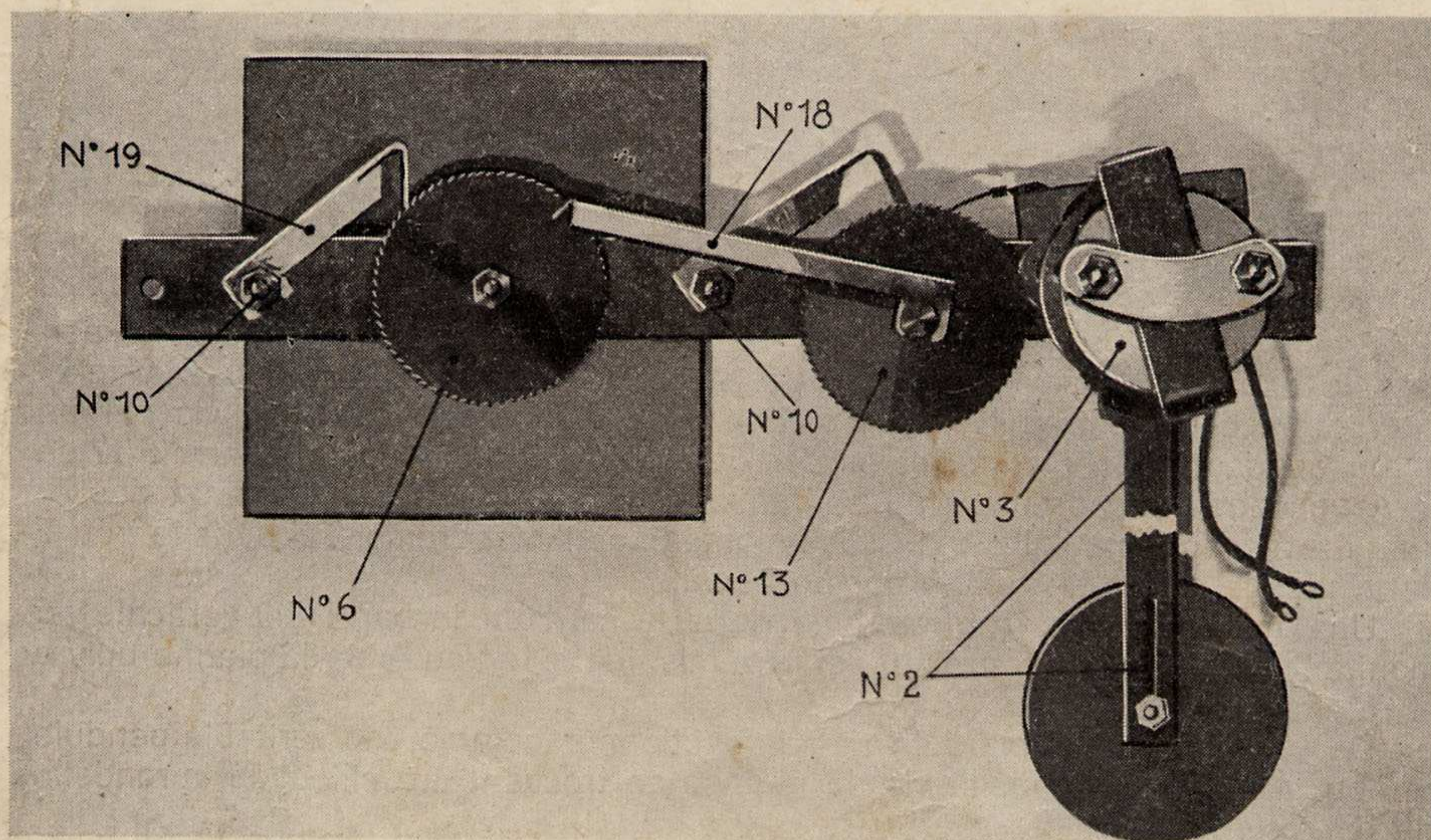
LA PARTIE HORLOGÈRE MONTÉE, VUE DE DERRIÈRE (N° 20)
