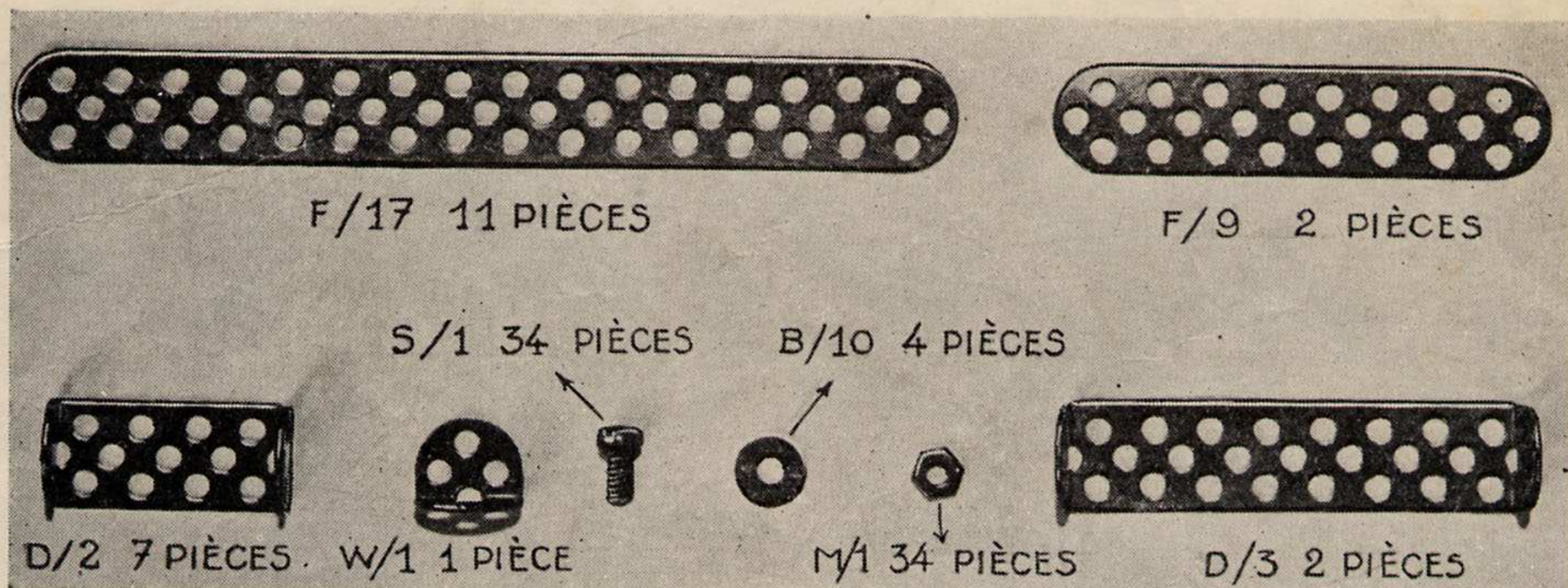
DÉTAIL DES PIÈCES DE CONSTRUCTION "TRIX"
