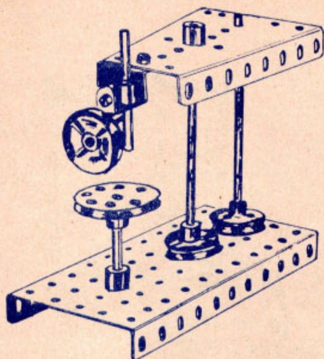
54 - Apparecchio per la durezza dei metalli
