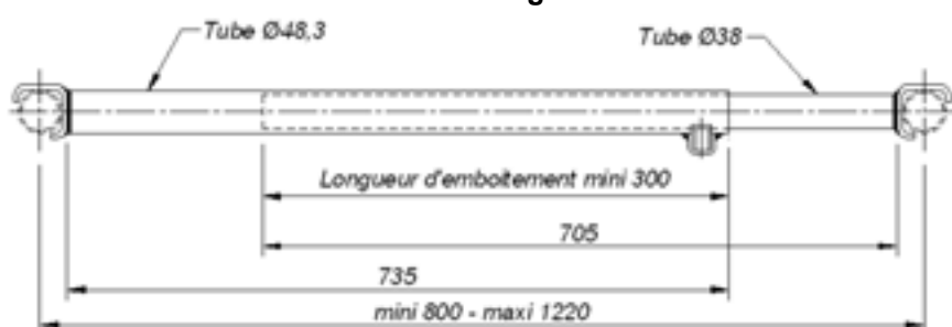
Traverse réglable
