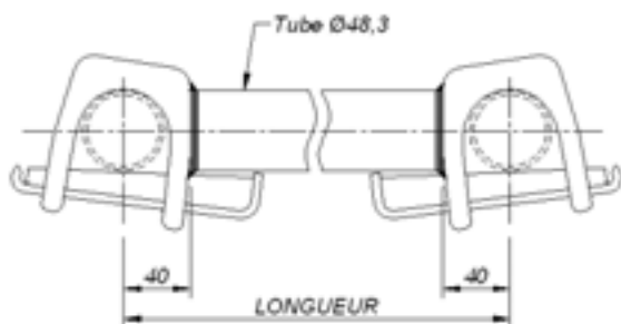
Traverse intermédiaire
