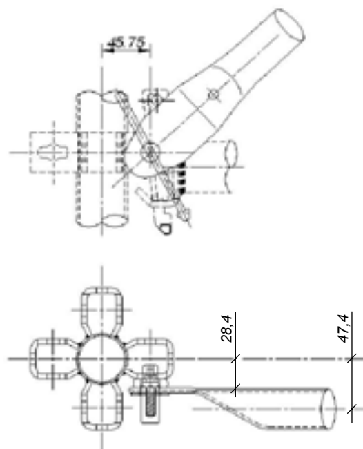
Montage avec diagonale
