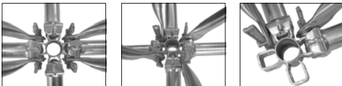
Montage avec moise
