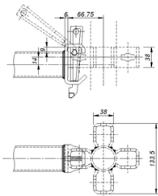
Montage avec moise
