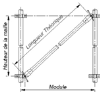
Longueur de la maille
