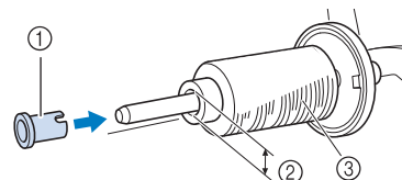
① Centre amovible pour bobine de fil (bobine de fil mini/très grande) ② Diamètre du trou de 8,0 mm à 10,5 mm (5/16"/pouce à 13/32"/pouce) ③ Bobine (fil bobiné de façon croisée)
