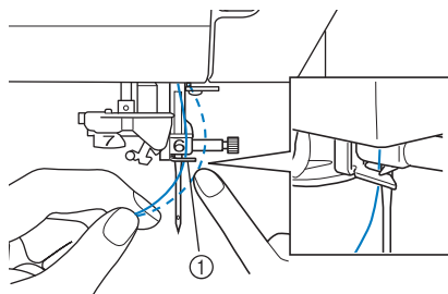
① Guide-fil de la barre de l'aiguille
